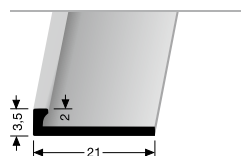
299 U KONCOVÝ PROFIL EDGE TRIM
