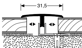
558 PŘECHODOVÝ PROFIL CONNECTING PROFILE
