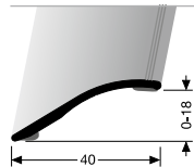
248 SK PROFIL NASTAVENÍ ADAPTING PROFILE
