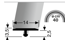
289 U T-PROFIL T-PROFILES
