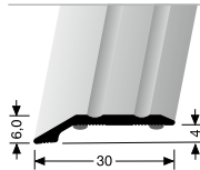
240 SK PROFIL NASTAVENÍ ADAPTING PROFILE
