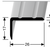
237 SK ÚHLOVÝ PROFIL ANGLE EDGE
