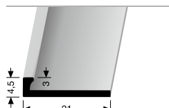
301 U KONCOVÝ PROFIL EDGE TRIM
