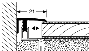
557 KONCOVÝ PROFIL BORDER PROFILE
