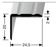
235 SK ÚHLOVÝ PROFIL ANGLE EDGE
