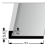
299 U KONCOVÝ PROFIL EDGE TRIM
