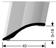
247 SK PROFIL NASTAVENÍ ADAPTING PROFILE
