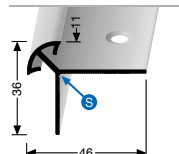
876 PROFIL SCHODIŠŤOVÉ LIŠTY STAIR NOSING
