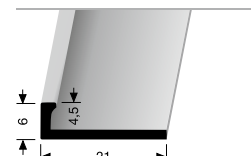
302 U KONCOVÝ PROFIL EDGE TRIM
