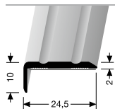
236 SK ÚHLOVÝ PROFIL ANGLE EDGE
