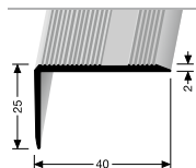
228 SK ÚHLOVÝ PROFIL ANGLE EDGE
