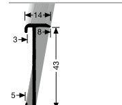
845 PROFIL SCHODIŠŤOVÉ LIŠTY STAIR NOSING
