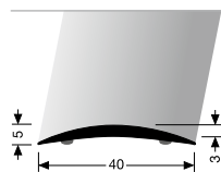
462 SK PŘECHODOVÝ PROFIL CONNECTING PROFILE
