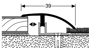
556 PROFIL NASTAVENÍ ADAPTING PROFILE
