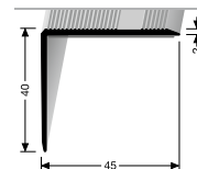
229 SK ÚHLOVÝ PROFIL ANGLE EDGE
