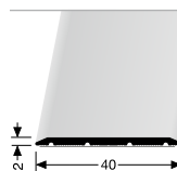
441 SK PŘECHODOVÝ PROFIL CONNECTING PROFILE
