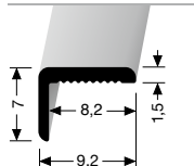
279 U ÚHLOVÝ PROFIL ANGLE EDGE
