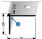
870 PROFIL SCHODIŠŤOVÉ LIŠTY STAIR NOSING
