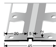
170 G KONEKTOR CONNECTOR
