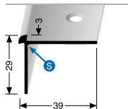
871 PROFIL SCHODIŠŤOVÉ LIŠTY STAIR NOSING
