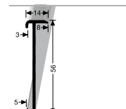
846 PROFIL SCHODIŠŤOVÉ LIŠTY STAIR NOSING
