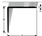
229 U ÚHLOVÝ PROFIL ANGLE EDGE
