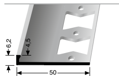
987 G PROFIL OKRAJOVÉHO SPOJE EDGE JOINT PROFILES
