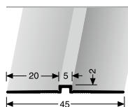
170 U KONEKTOR CONNECTOR
