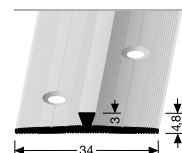
365 KONCOVÝ PROFIL EDGE TRIM
