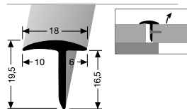
294 PROFIL HRANY EDGE TRIM
