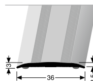
440 SK PŘECHODOVÝ PROFIL CONNECTING PROFILE
