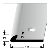
355 KONCOVÝ PROFIL EDGE TRIM
