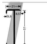
847 PROFIL SCHODIŠŤOVÉ LIŠTY STAIR NOSING
