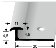
345 PROFIL HRANY EDGE TRIM
