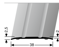
438 SK PŘECHODOVÝ PROFIL CONNECTING PROFILE
