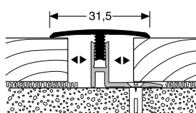
561 PŘECHODOVÝ PROFIL CONNECTING PROFILE
