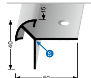
879 PROFIL SCHODIŠŤOVÉ LIŠTY STAIR NOSING
