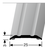
230 SK PŘECHODOVÝ PROFIL CONNECTING PROFILE
