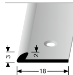
355 KONCOVÝ PROFIL BORDER PROFILE
