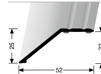
245 SK PROFIL NASTAVENÍ ADAPTING PROFILE
