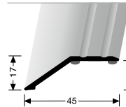
241 SK PROFIL NASTAVENÍ ADAPTING PROFILE
