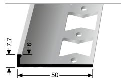
988 G PROFIL OKRAJOVÉHO SPOJE EDGE JOINT PROFILES
