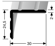
234 SK ÚHLOVÝ PROFIL ANGLE EDGE
