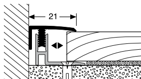
560 KONCOVÝ PROFIL BORDER PROFILE
