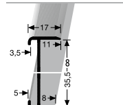
844 WS PROFIL SCHODIŠŤOVÉ LIŠTY STAIR NOSING
