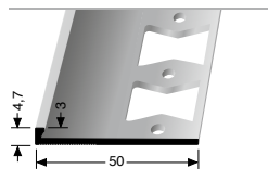
986 G PROFIL OKRAJOVÉHO SPOJE EDGE JOINT PROFILES
