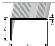
228 U ÚHLOVÝ PROFIL ANGLE EDGE
