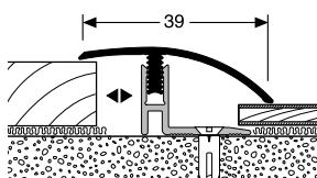
559 PROFIL NASTAVENÍ ADAPTING PROFILE
